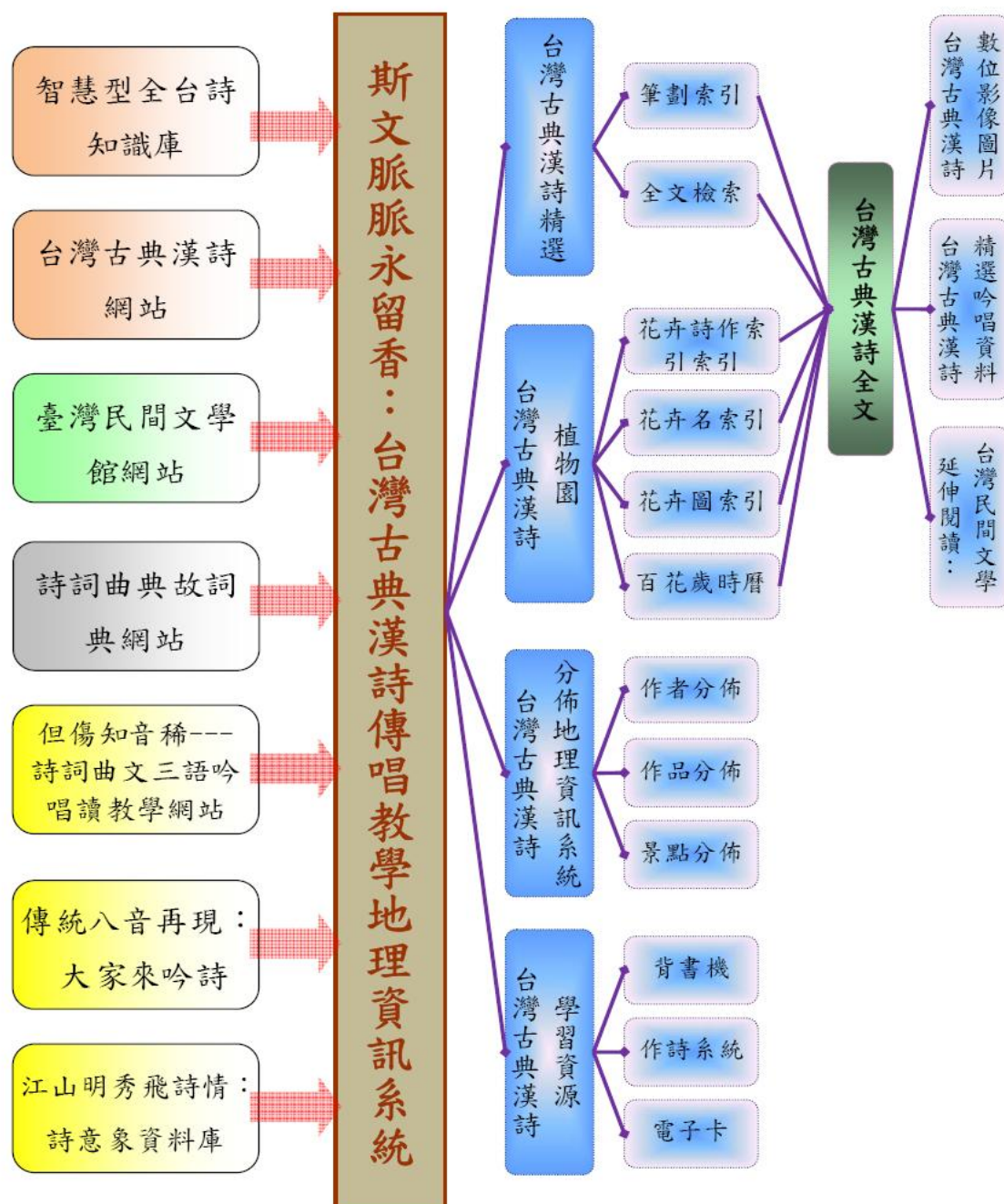
斯文脈脈永留香：台灣古典漢詩傳唱教學地理資訊系統網站架構圖
